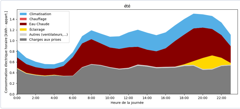
Profil de consommation journalière moyen des jours d'hiver et d'été, montrant la contribution du chauffage, de l'éclairage, de l'eau chaude sanitaire, des charges aux prises et des systèmes auxiliaires au cours d'une journée hivernale ou estivale moyenne.
